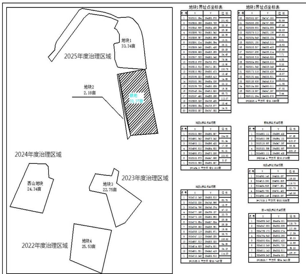
2022 年--2025 年突泉县太平红瑞采石有限公司矿山地质环境治 理与土地复垦工作部署图
